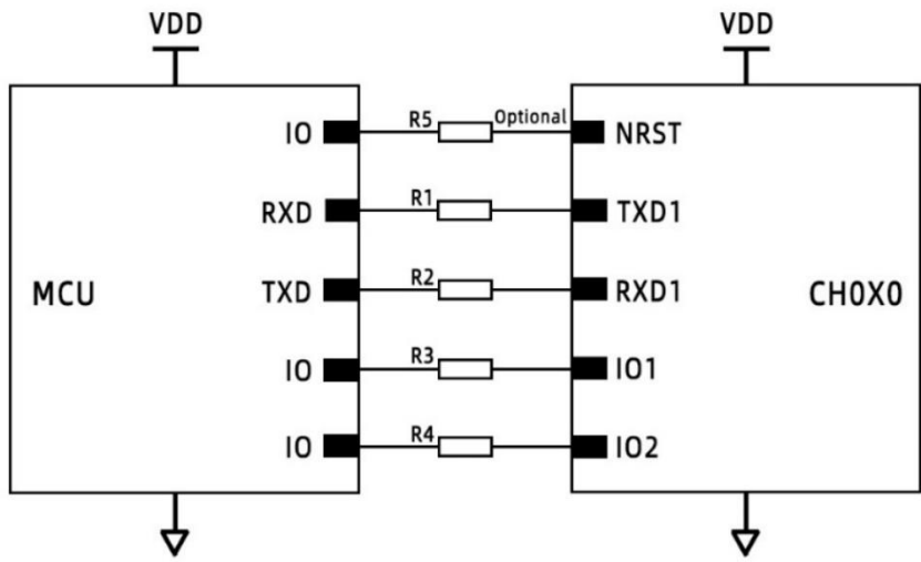
Figure19: CH0X0 串口通信不带同步
