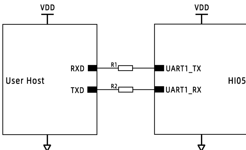
Figure6: HI05 串口通信参考电路
