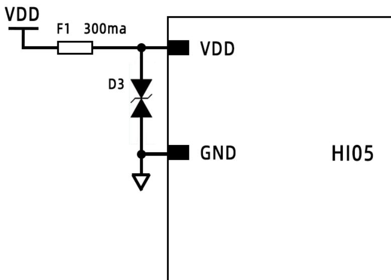
Figure5: HI05 电源参考电路
