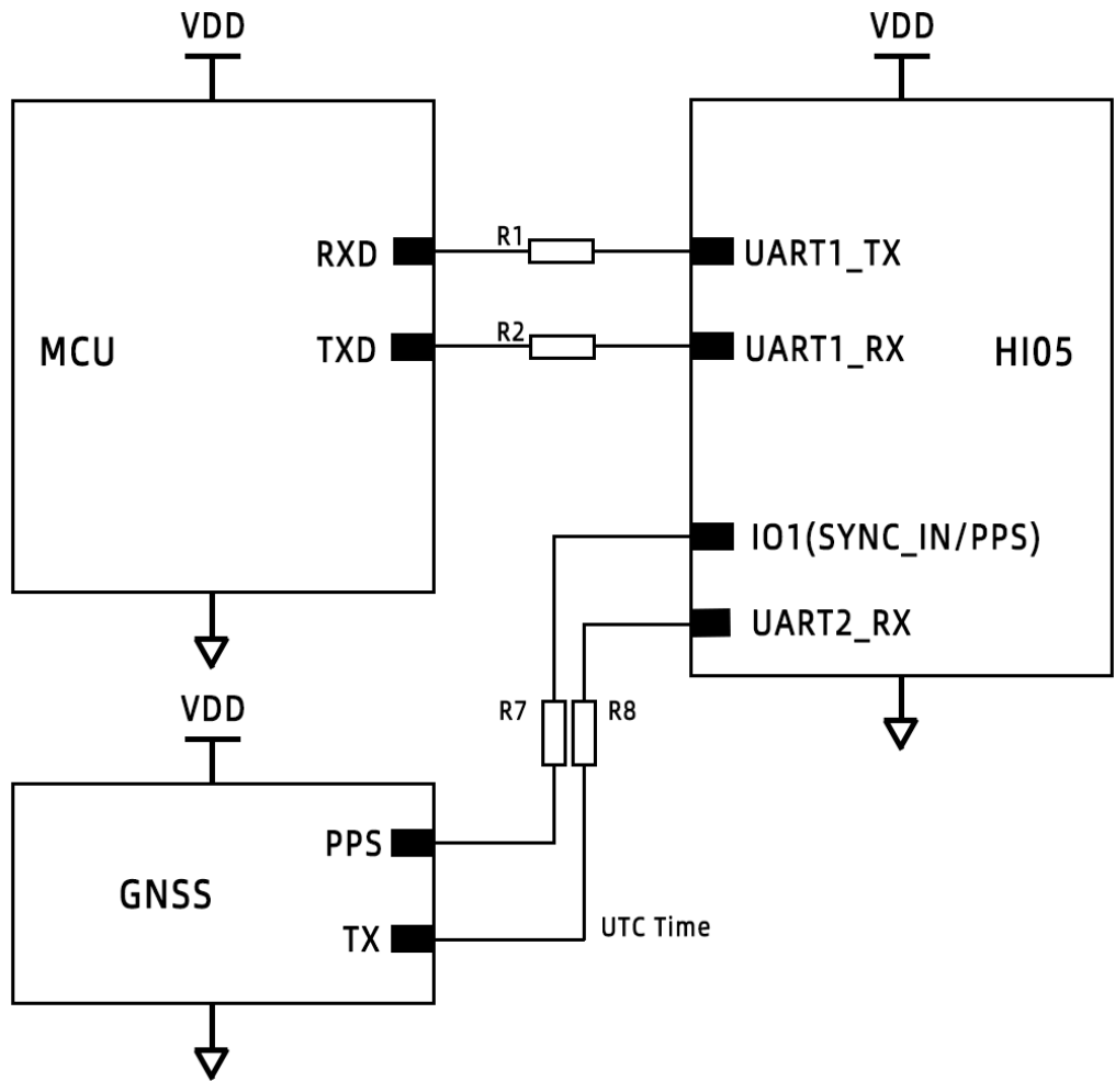
Figure10: HI05 与 GNSS 同步
