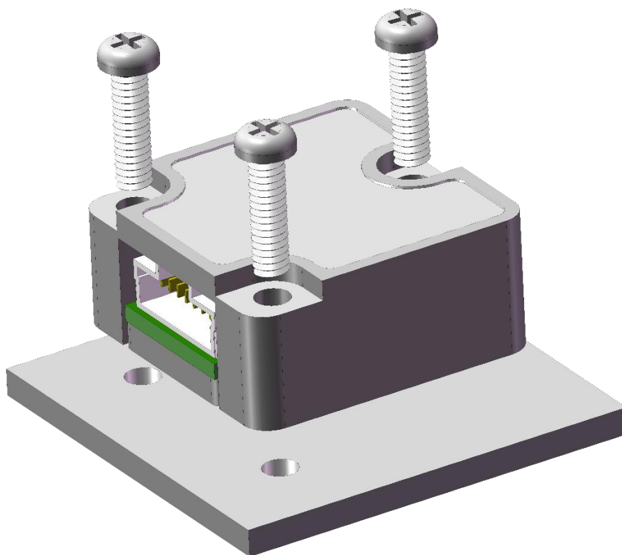
图 12: 安装示意图
