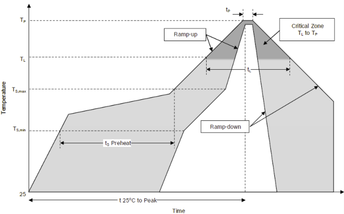
Figure21: SMT 温度曲线
